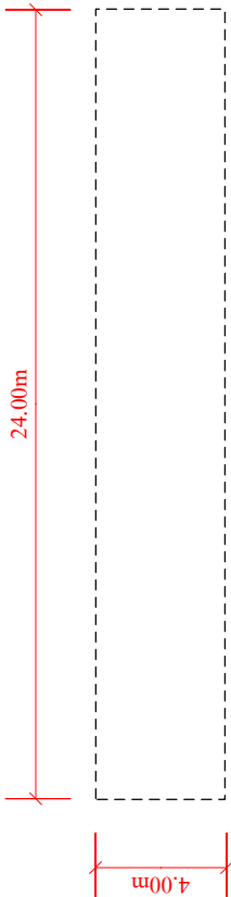
สิ่งปลูกสร้างรายการที่ 3.10 / ที่จอดรถยนต์ (หลังคาคลุม) หลังที่ 20
